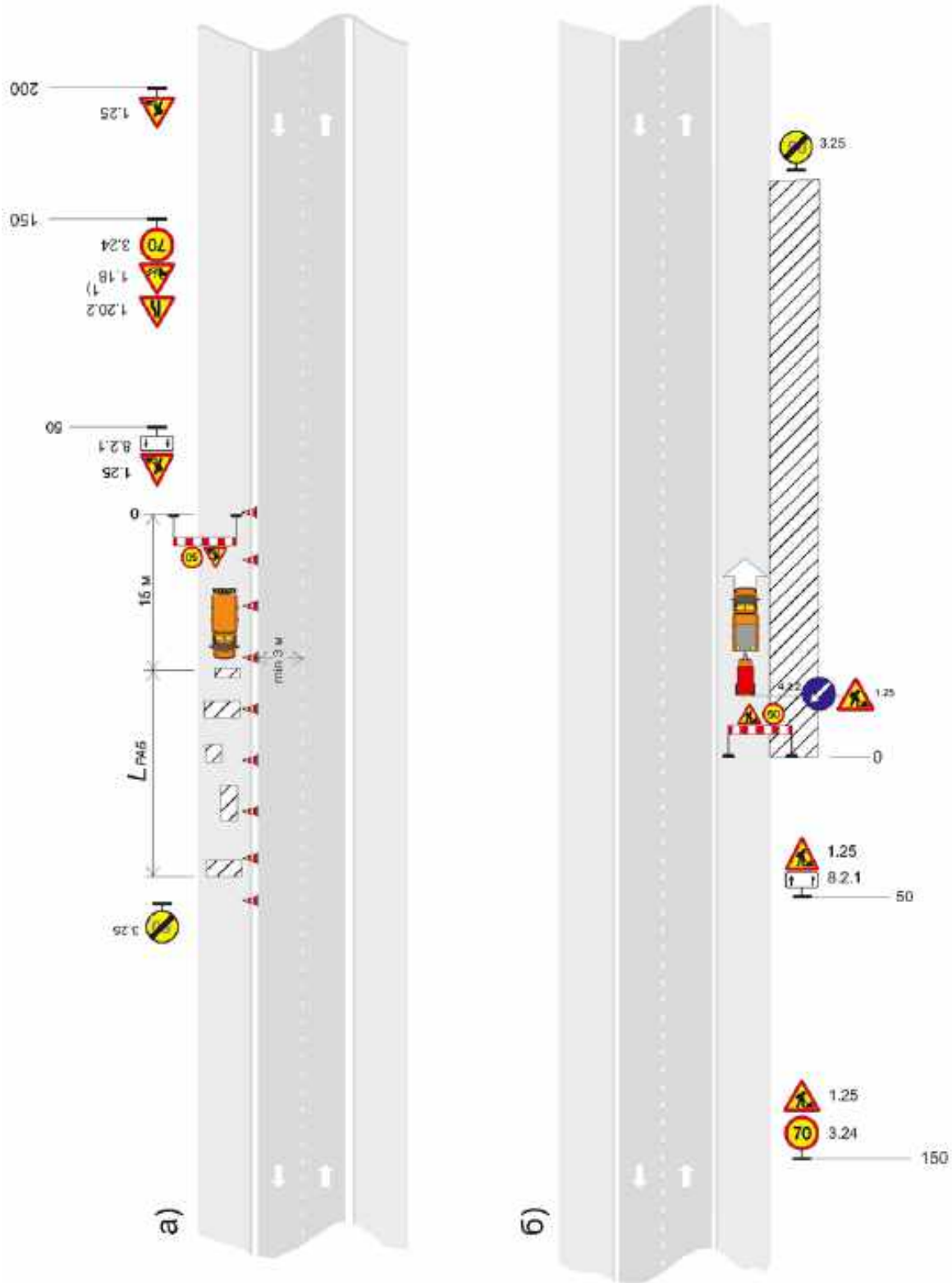
1) - знак устанавливают перед участками дорог, на которых возможен выброс гравия, щебня и т.п. из-под колес транспортных средств
