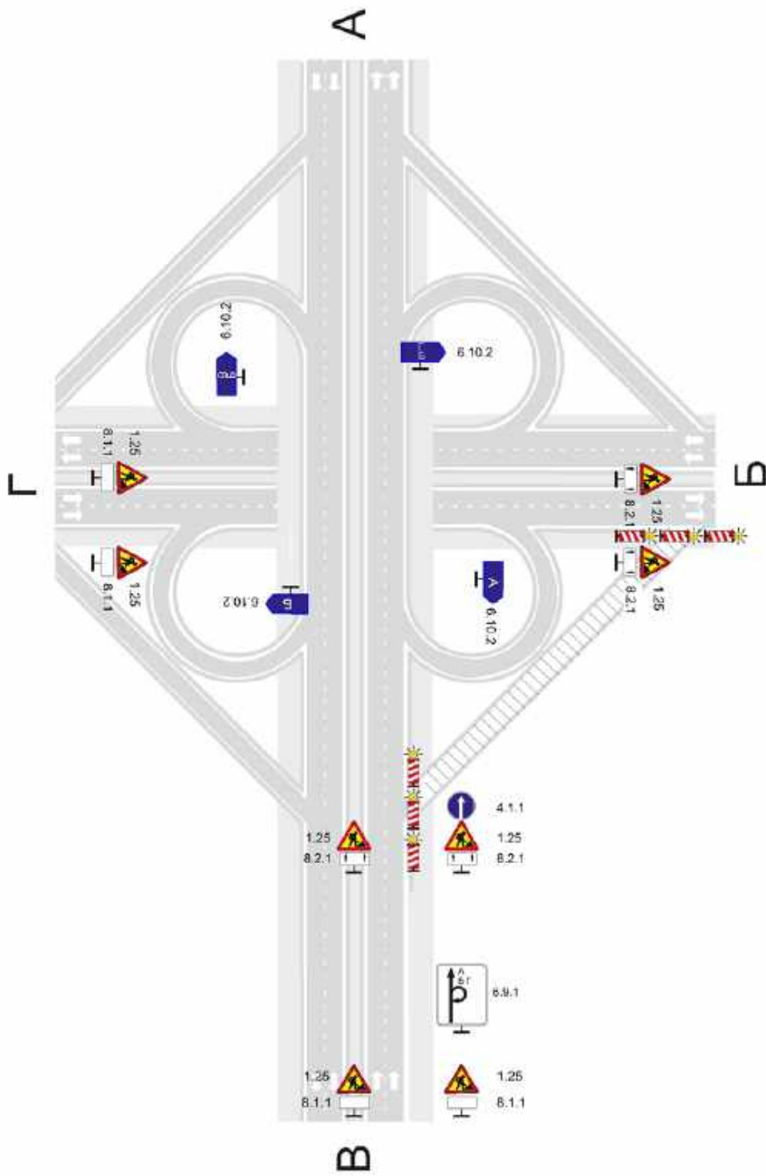
Рисунок Б.32 – Транспортная развязка - клеверный лист. Зона производства работ на правооборотном съезде. Пропуск транспортных средств по левооборотным съездам
