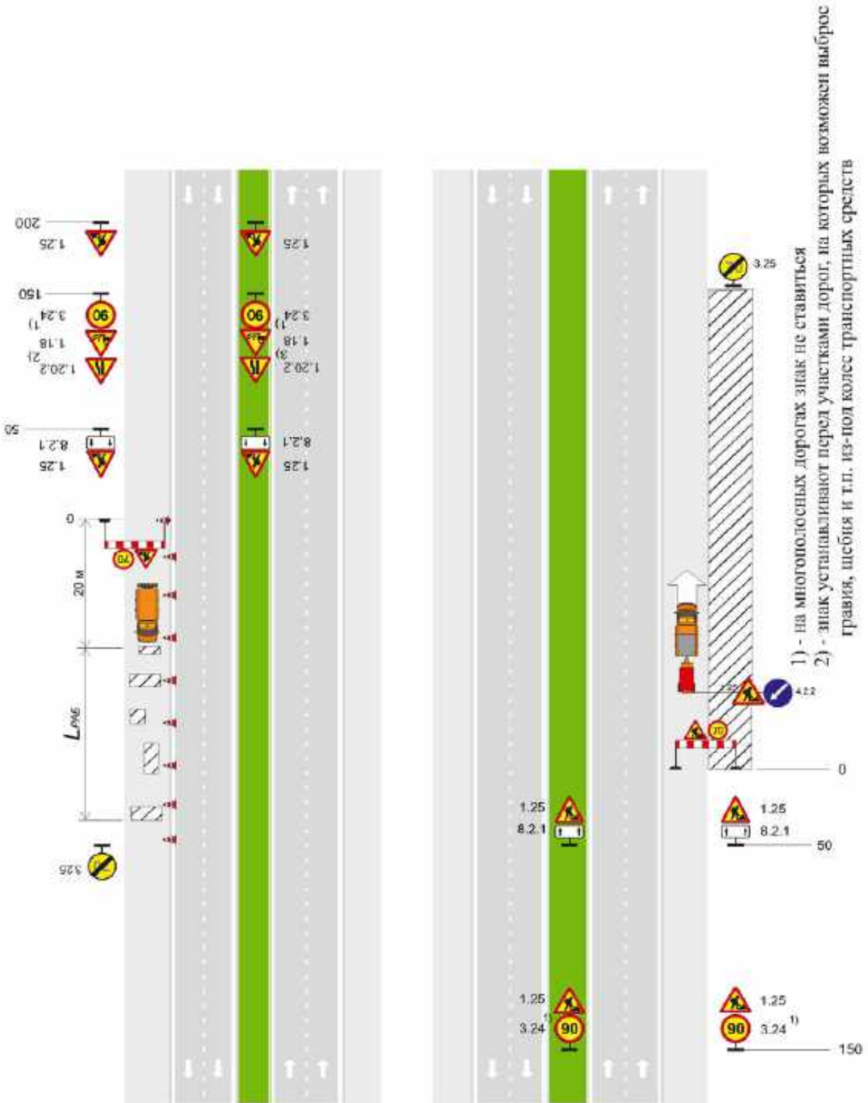
Рисунок Б.37 - Автомагистраль, скоростная дорога, многополосная дорога обычного типа. Рабочая зона краскосерочных работ на обочине или откосе
